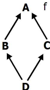
Figura 4.8: Herencia múltiple y herencia repetida
