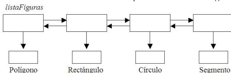
Figura 4.3: Ejemplo de estructura de datos polimorfa
